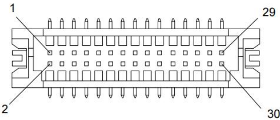
2*15PIN_1.25mm 间距 180 度
